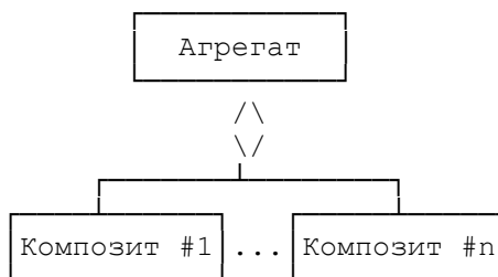
Рисунок А.4. Отношение агрегирования между UML-классами
