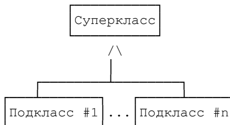
Рисунок А.5. Отношение обобщения между UML-классами
