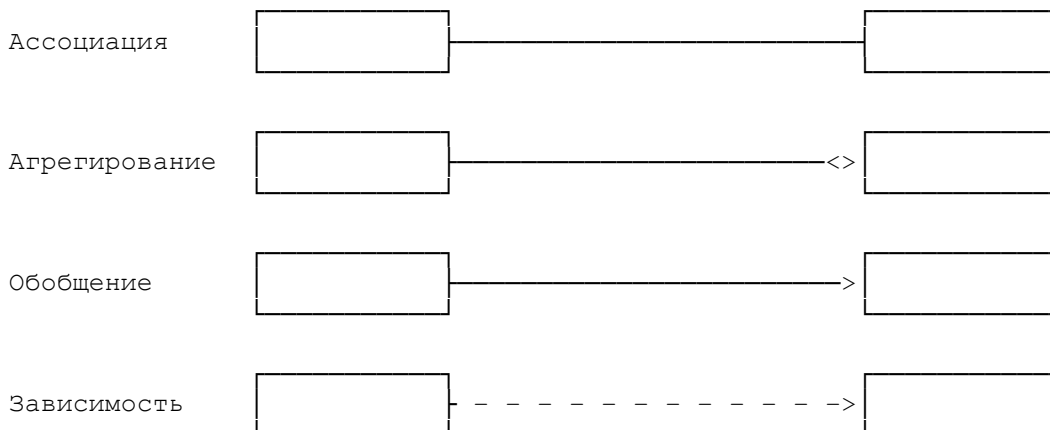
Рисунок А.1. Основные виды отношений UML
