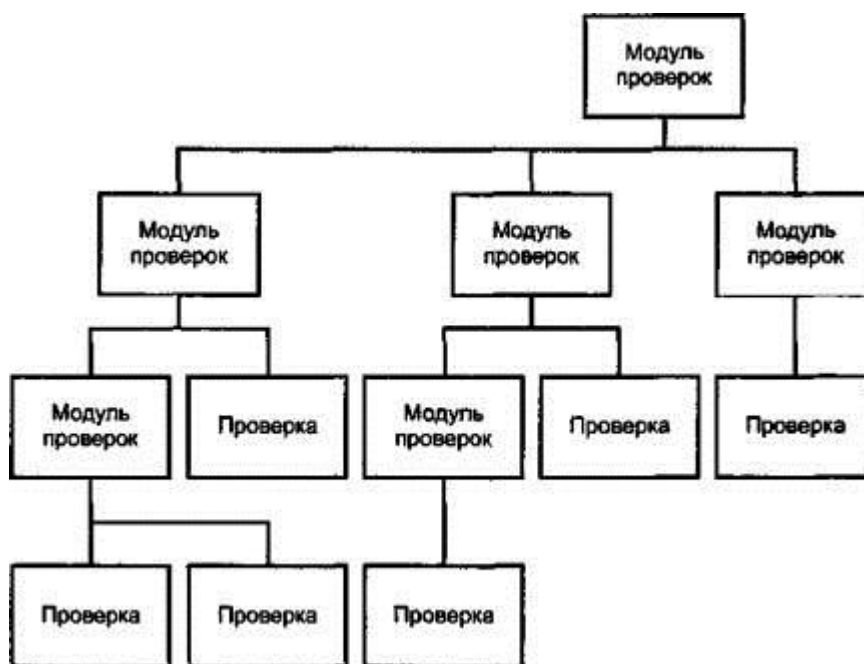
Рисунок 2 - Пример иерархической структуры КИ
